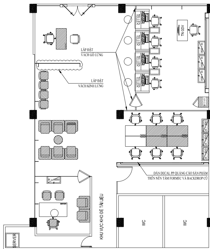
MẶT BẰNG CẢI TẠO
