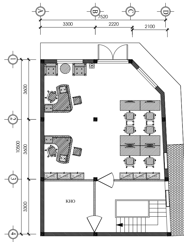
MẶT BẰNG CẢI TẠO
