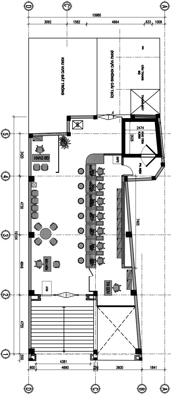
MẶT BẰNG NỘI THẤT TẦNG 1
